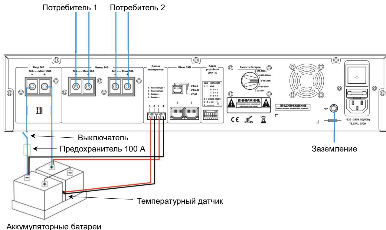
Рис. 4.1. Схема внешних подключений резервного источника питания и зарядного устройства LPA-EVA-BC
